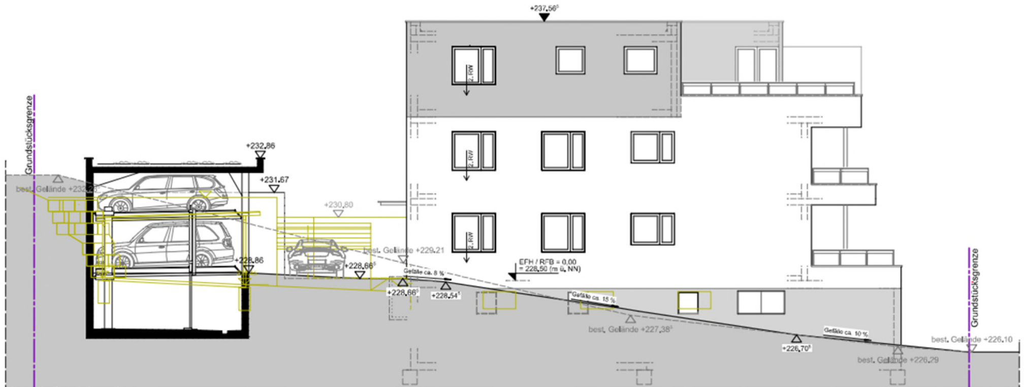
Ansicht Nord
