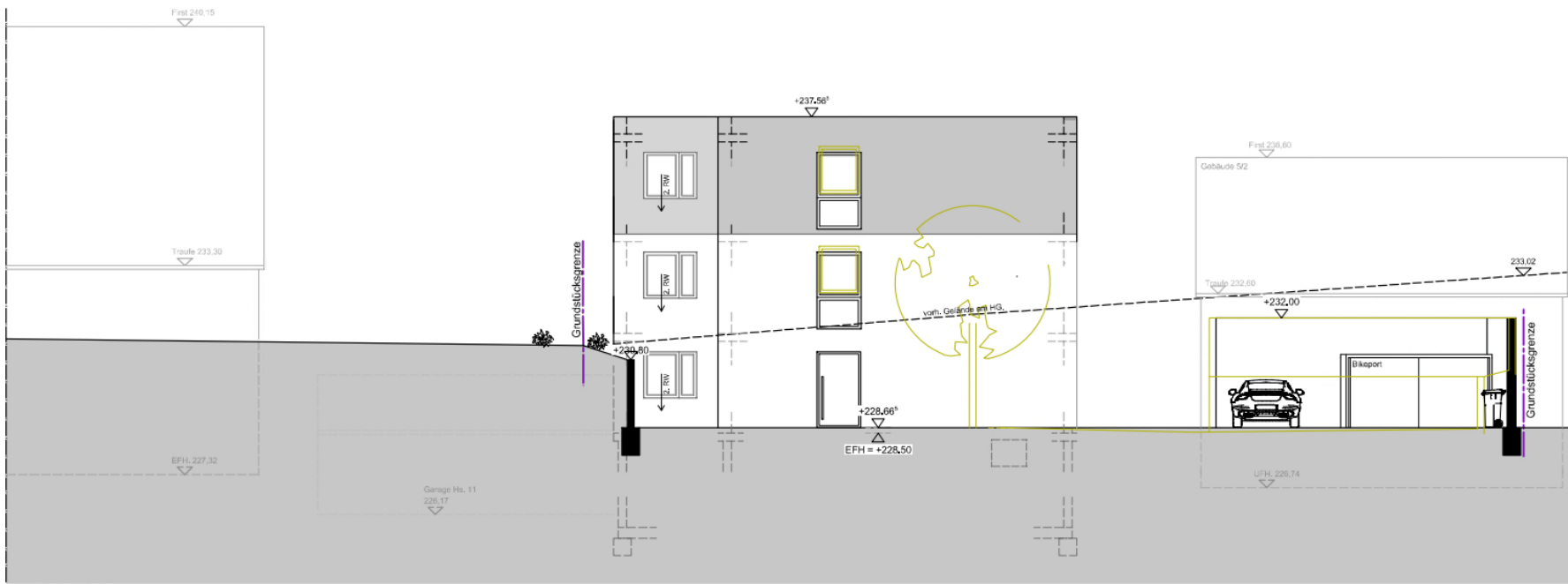
Ansicht Ost
