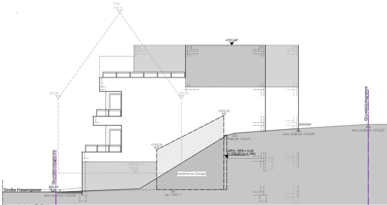
Ansicht Süd
